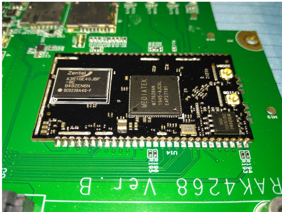
Wi-Fi IC
