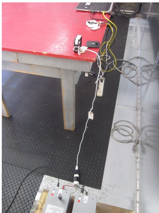
EUT Configuration
