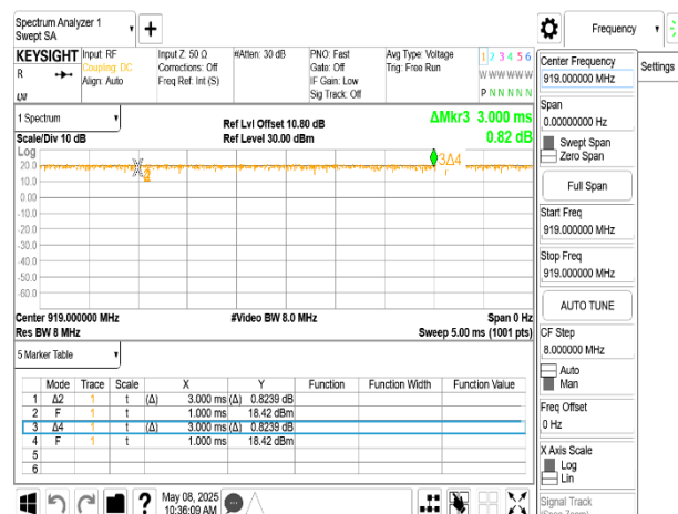
OFDM_2M_919MHz
