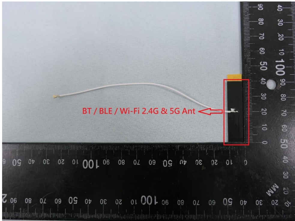
(12) PCB Antenna
