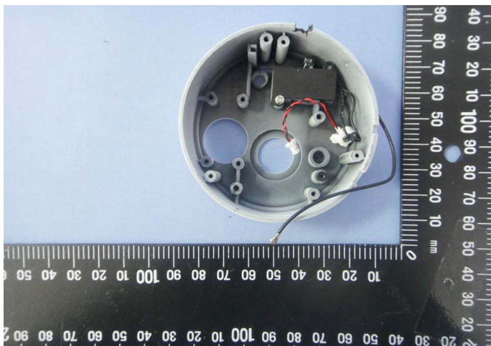
EUT Photo 18 )
