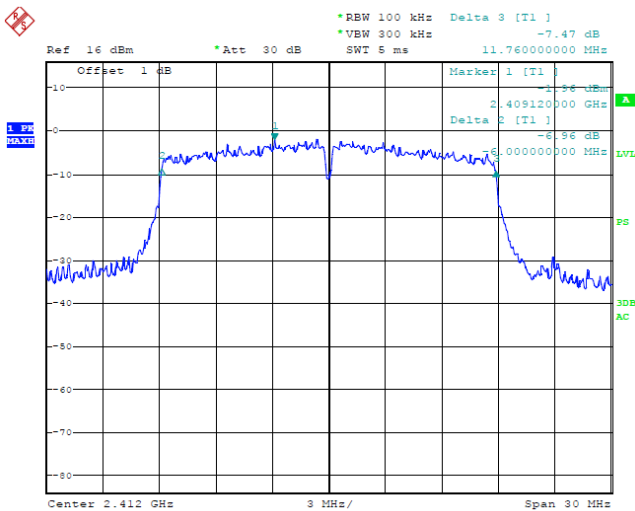
CH1 / 2412 MHz
