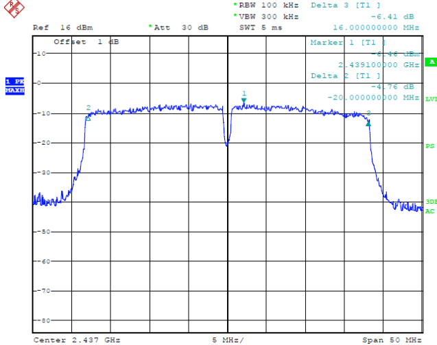
CH6 / 2437 MHz
