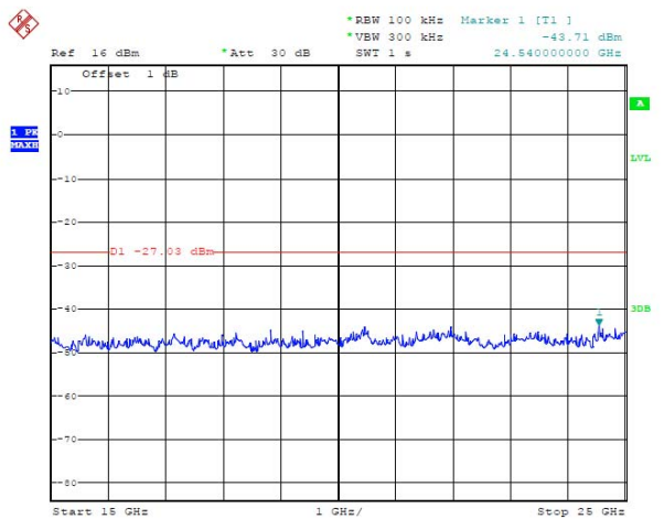
15GHz~25GHz
