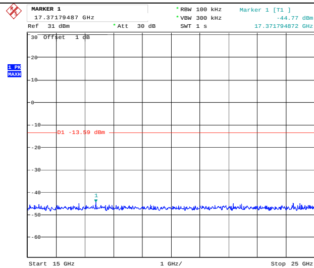
15GHz-25GHz
