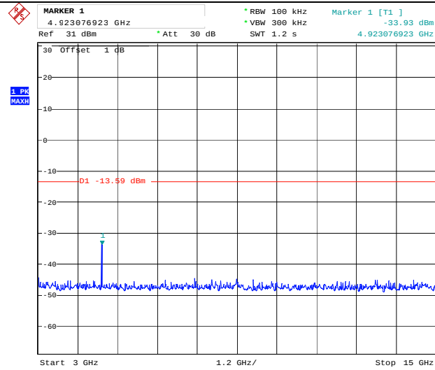
3GHz-15GHz
