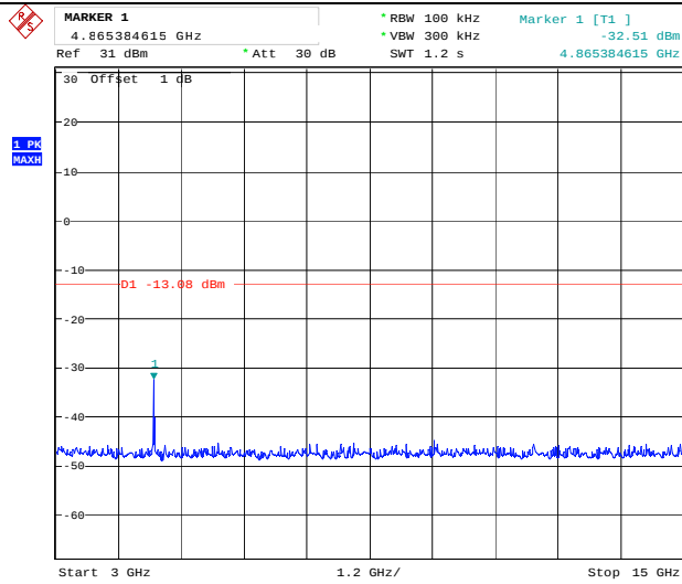
3GHz-15GHz
