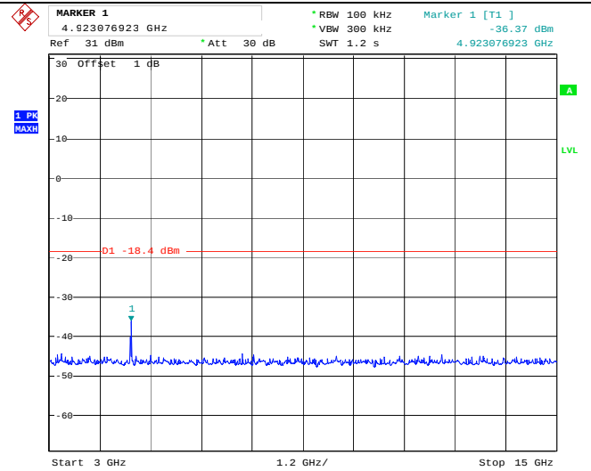
3GHz-15GHz
