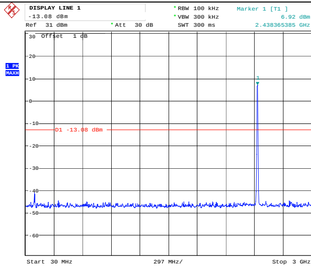
30MHz-3GHz
