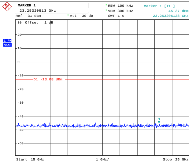
15GHz-25GHz
