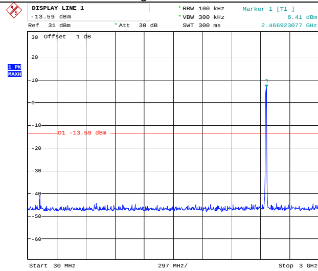
30MHz-3GHz
