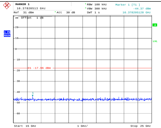
15GHz-25GHz
