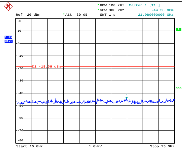
15GHz-25GHz
