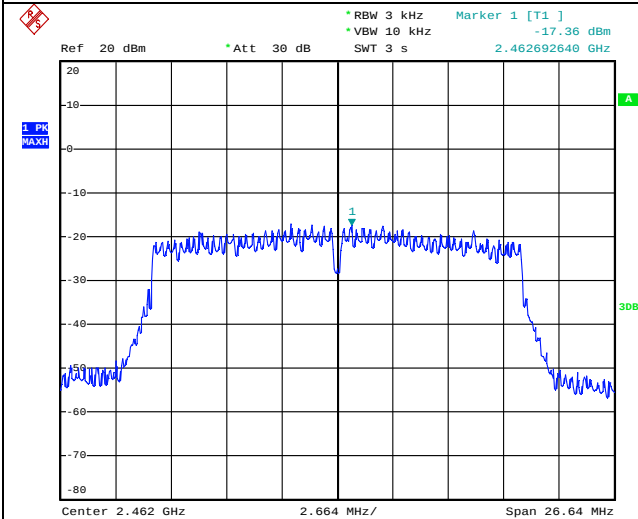
2462 MHz
