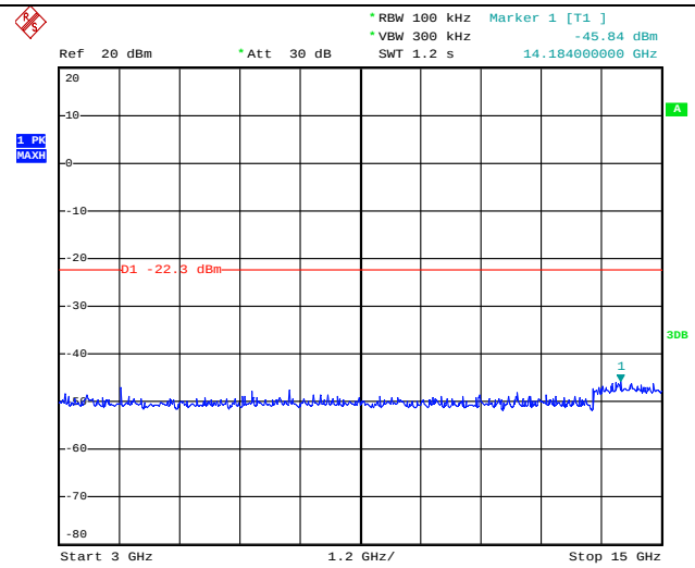
3GHz-15GHz
