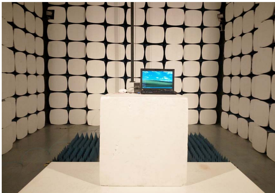
Above 1GHz:
