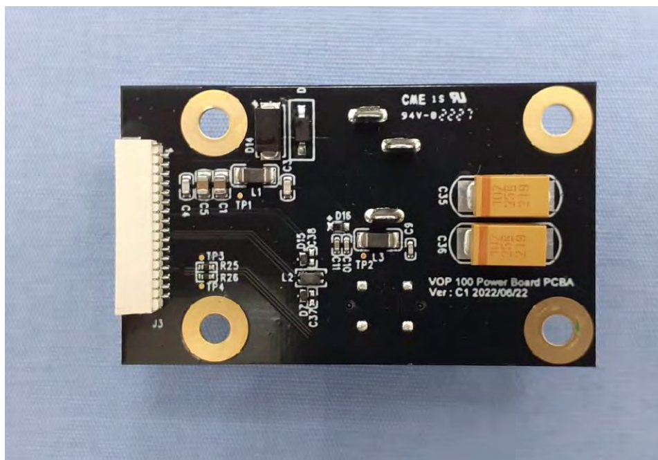
EUT Photo (54)
