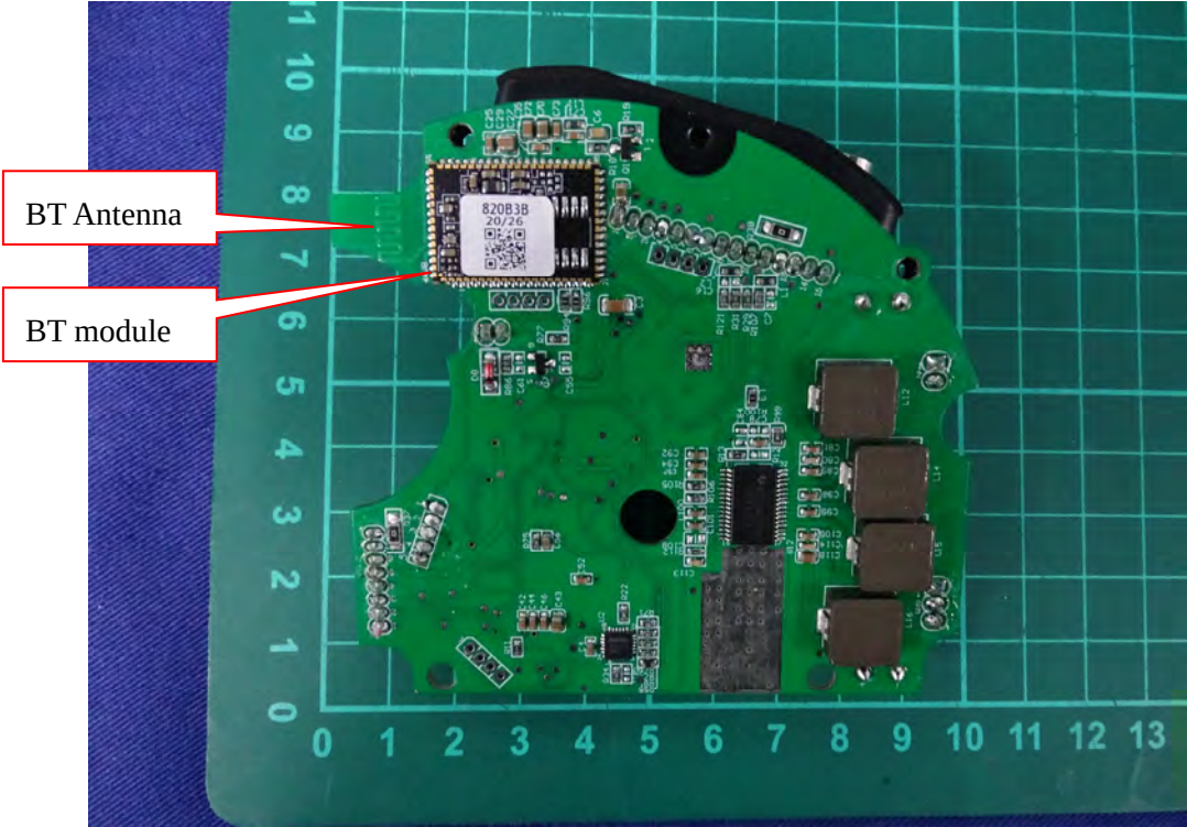
(14) EUT Photo
