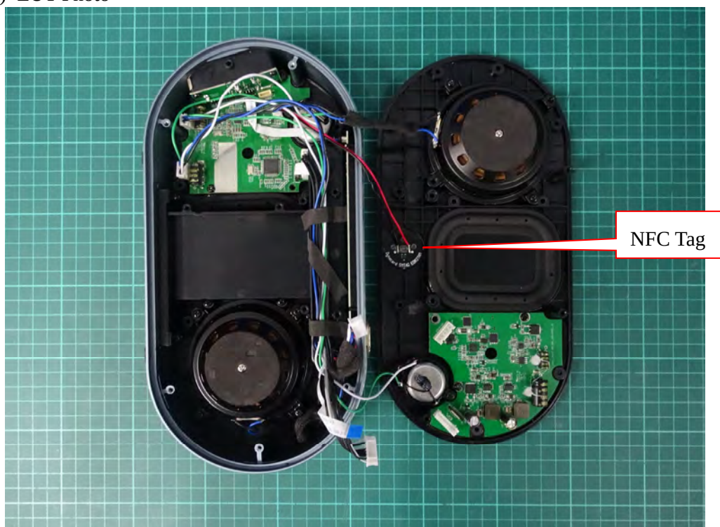
(12) EUT Photo
