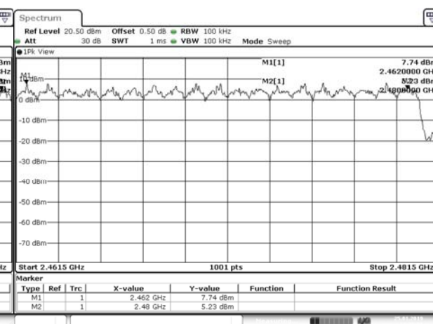
2462-2480MHz
