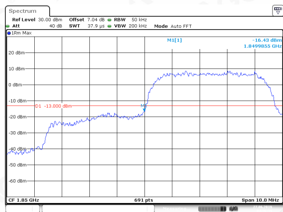
WCDMA 1900-LCH
