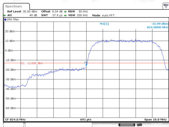
WCDMA 850-LCH
