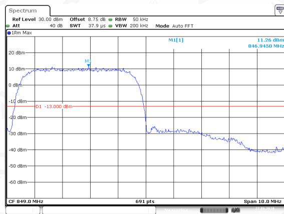
WCDMA 850-HCH
