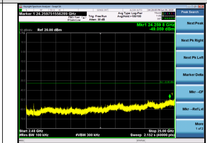
11nHT40-LCH
