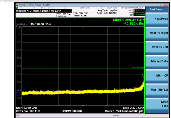
11nHT40-LCH
