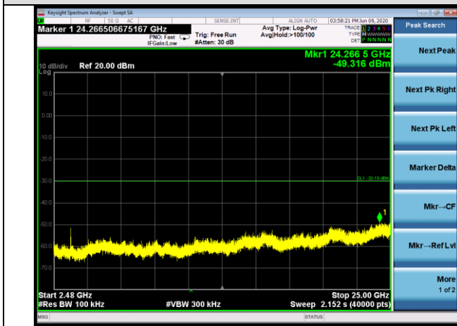
11nHT20-LCH
