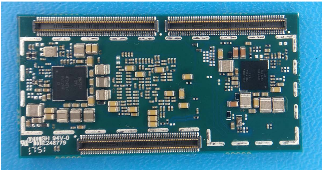
Bottom Side
