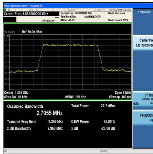
Band2-3MHz-QPSK-18615-15RB#0-2.7055
