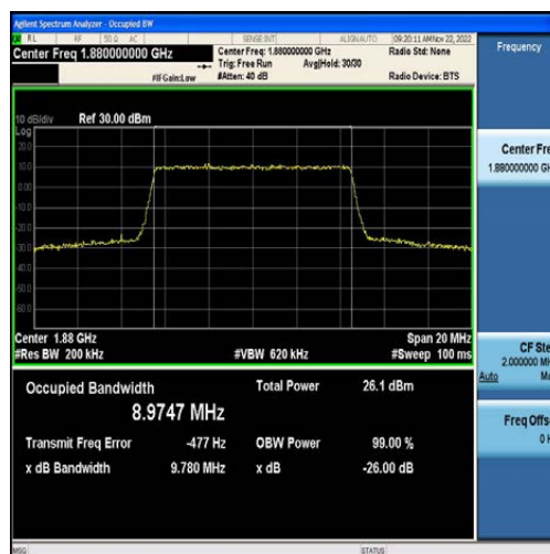
Band2-10MHz-QPSK-18900-50RB#0-8.9747
