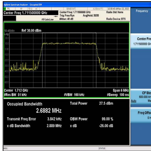
Band4-3MHz-QPSK-19965-15RB#0-2.6882
