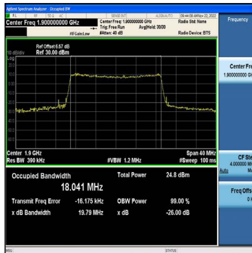
Band2-20MHz-QPSK-19100-100RB#0-18.041
