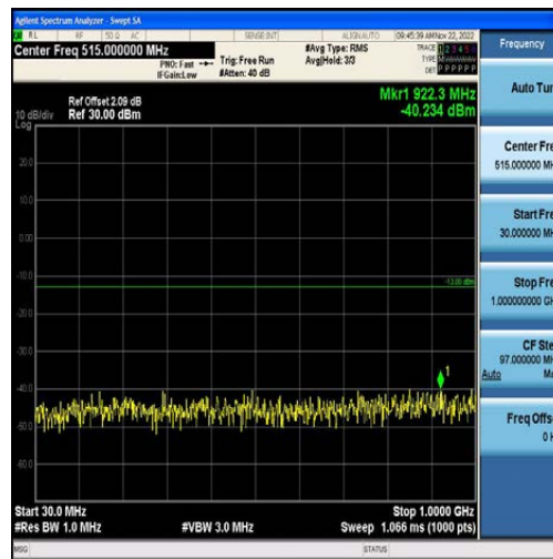
Band2-20MHz-QPSK-18700-100RB#0-Range1:30~1000MHz
