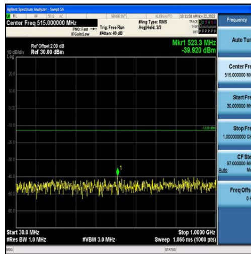
Band4-3MHz-QPSK-19965-15RB#0-Range1:30~1000MHz
