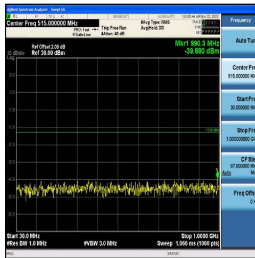
Band4-1.4MHz-QPSK-19957-6RB#0-Range1:30~1000MHz
