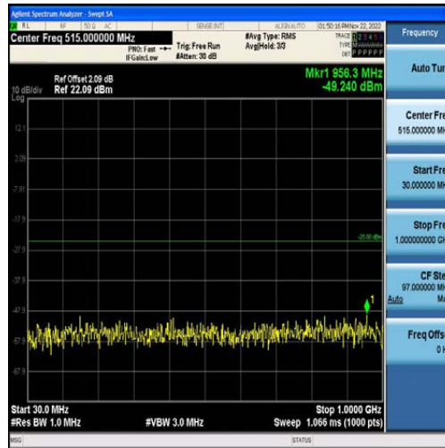
Band7-10MHz-QPSK-20800-50RB#0-Range1:30~1000MHz
