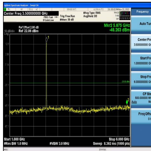
Band7-5MHz-QPSK-21100-25RB#0-Range2:1000~6000MHz
