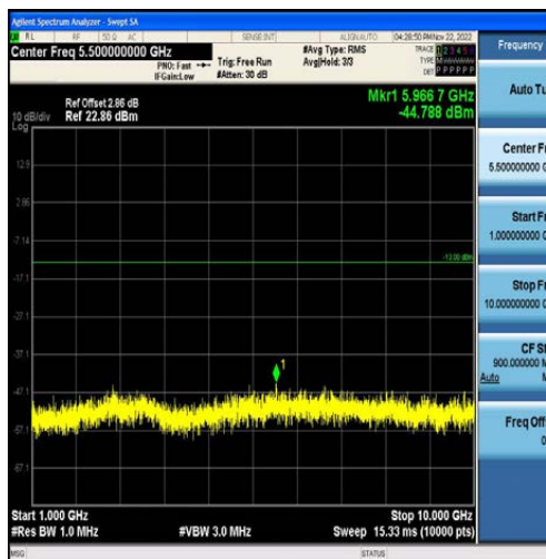
Band13-5MHz-QPSK-23230-25RB#0-Range2:1000~10000MHz
