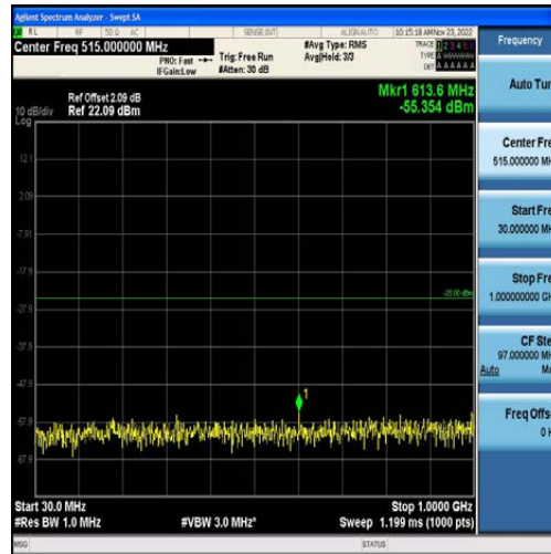
Band41-10MHz-QPSK-39700-50RB#0-Range1:30~1000MHz
