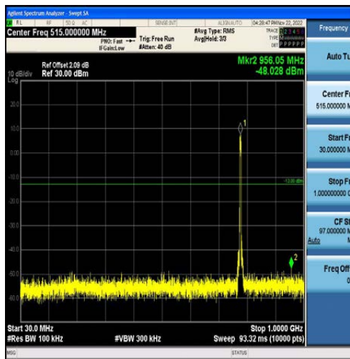
Band13-5MHz-QPSK-23230-25RB#0-Range1:30~1000MHz
