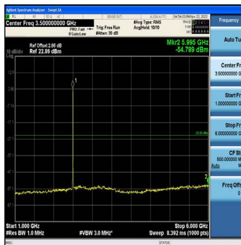
Band41-5MHz-QPSK-39675-25RB#0-Range2:1000~6000MHz
