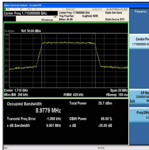
Band4-10MHz-QPSK-20000-50RB#0-8.9779
