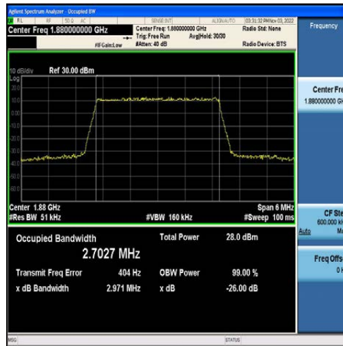
Band2-3MHz-QPSK-18900-15RB#0-2.7027
