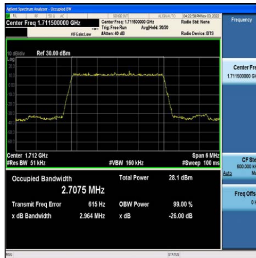
Band4-3MHz-QPSK-19965-15RB#0-2.7075
