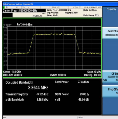
Band2-10MHz-16QAM-18900-50RB#0-8.9544
