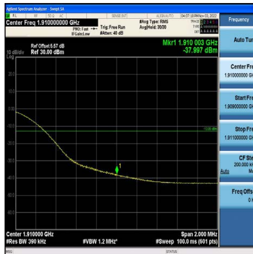
Band2-20MHz-QPSK-19100-100RB#0
