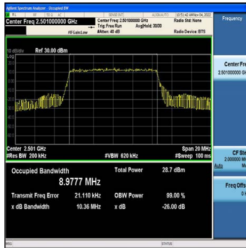
Band41-10MHz-QPSK-39700-50RB#0-8.9777
