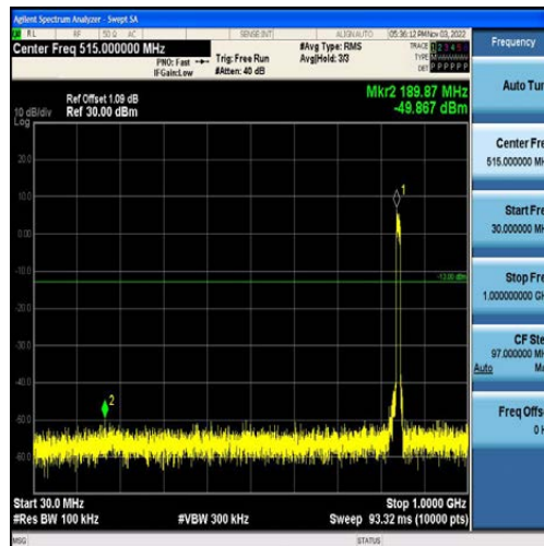
Band5-10MHz-QPSK-20600-50RB#0-Range1:30~1000MHz
