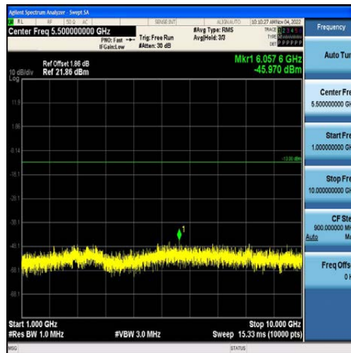
Band12-10MHz-QPSK-23130-50RB#0-Range2:1000~10000MHz
