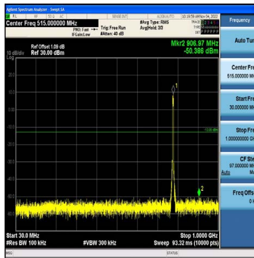
Band13-5MHz-QPSK-23230-25RB#0-Range1:30~1000MHz
