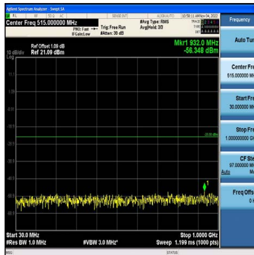
Band41-10MHz-QPSK-41540-50RB#0-Range1:30~1000MHz
