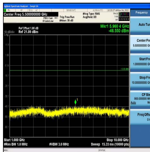
Band13-5MHz-QPSK-23255-25RB#0-Range2:1000~10000MHz
