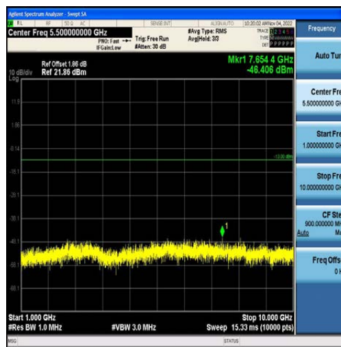
Band13-5MHz-QPSK-23230-25RB#0-Range2:1000~10000MHz
