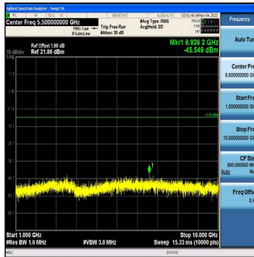
Band12-5MHz-QPSK-23095-25RB#0-Range2:1000~10000MHz
