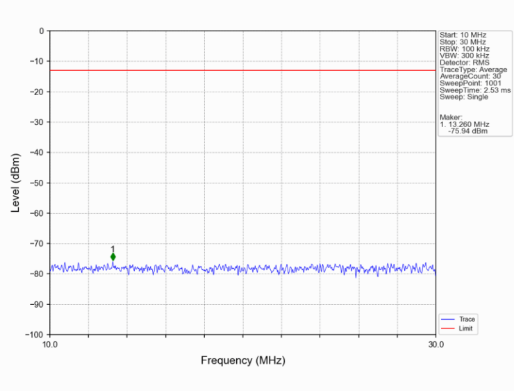
Band12 1.4MHz QPSK MCH 707.5MHz RB 1 0 NTV
