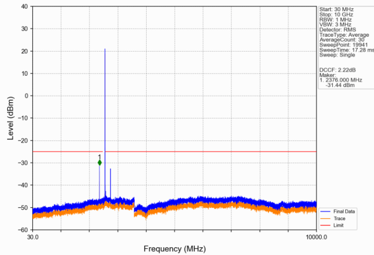
Band38 5MHz QPSK LCH 2572.5MHz RB 1 0 NTV
