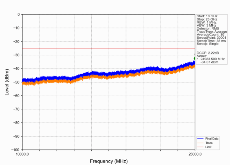
Band38 10MHz QPSK HCH 2615MHz RB 1 0 NTNV
