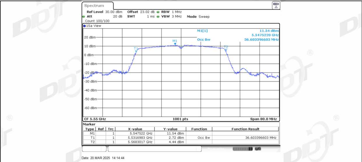
11AC40MIMO_Ant2_5550
