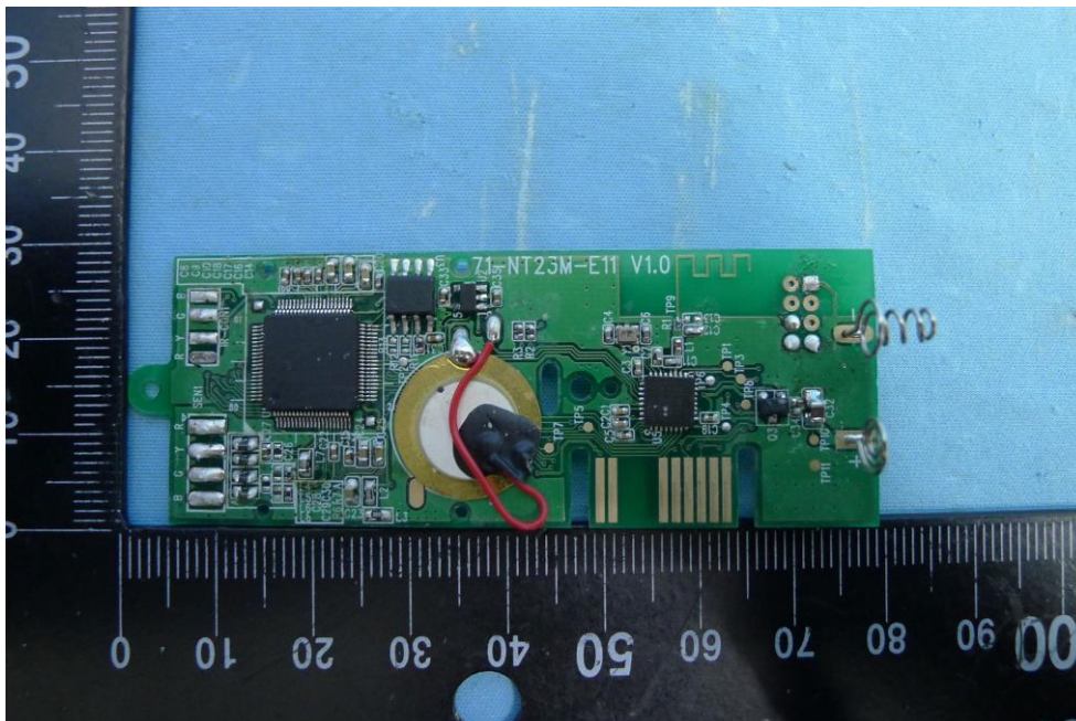
(8) EUT Photo
