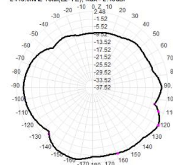
2440.0MHz Total(E2-YZ), Max= 2.48dBi
