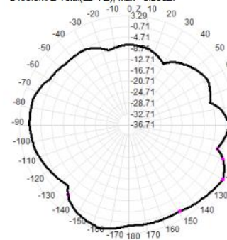
2485.0MHz Total(E2-YZ), Max= 3.37dBi
