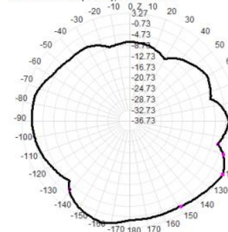
2475.0MHz Total(E2-YZ), Max= 3.27dBi
