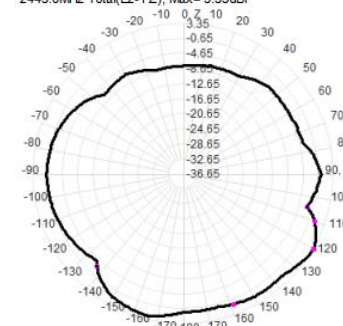
2445.0MHz Total(E2-YZ), Max= 3.35dBi
