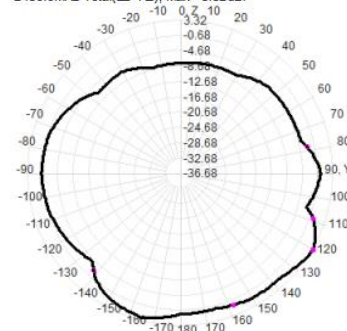
2450.0MHz Total(E2-YZ), Max= 3.32dBi
