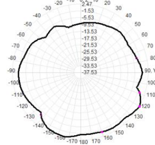
2415.0MHz Total(E2-YZ), Max= 2.47dBi
