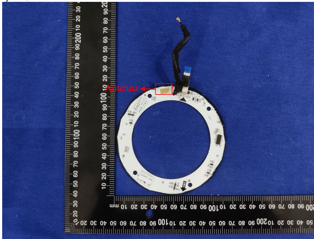
8) EUT Photo
