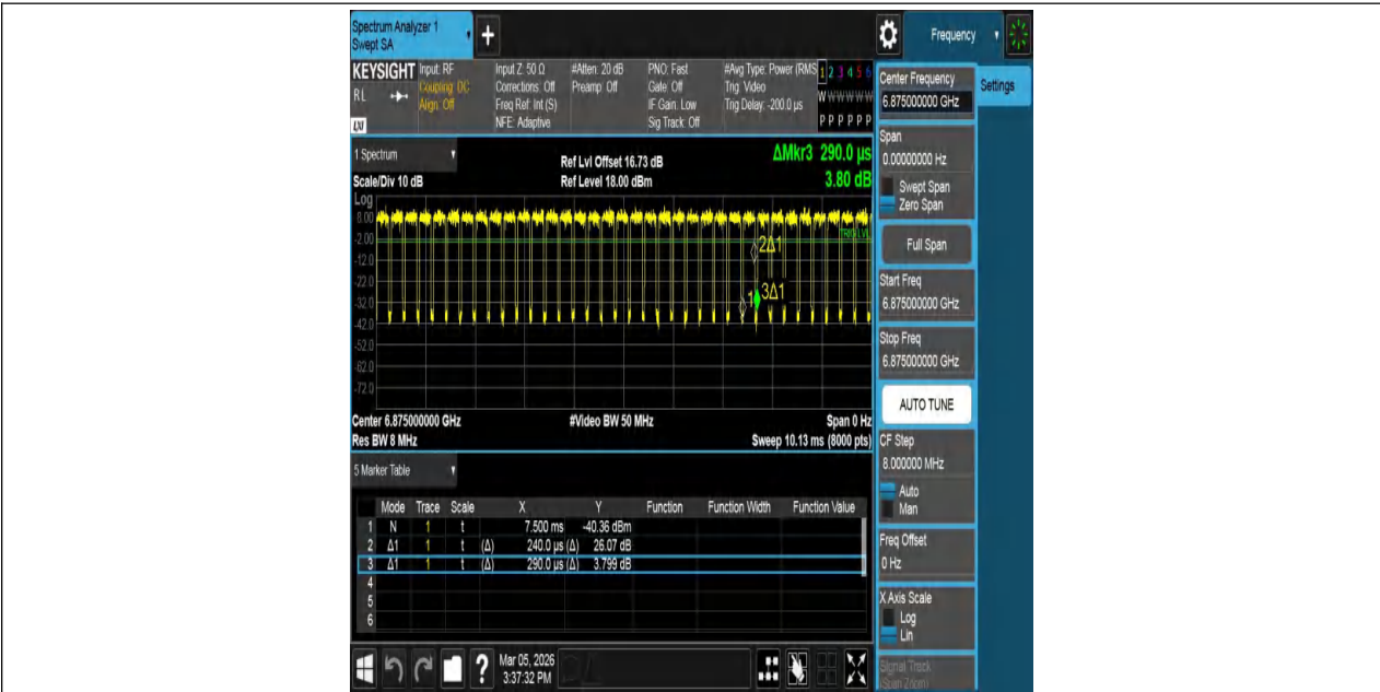
NTNV-11BE20MIMO-Ant1-6875
