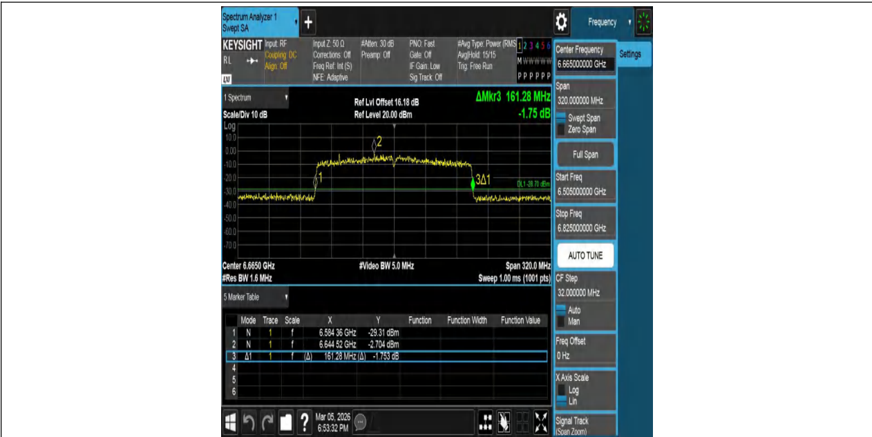
11BE160MIMO-Ant1-6665
