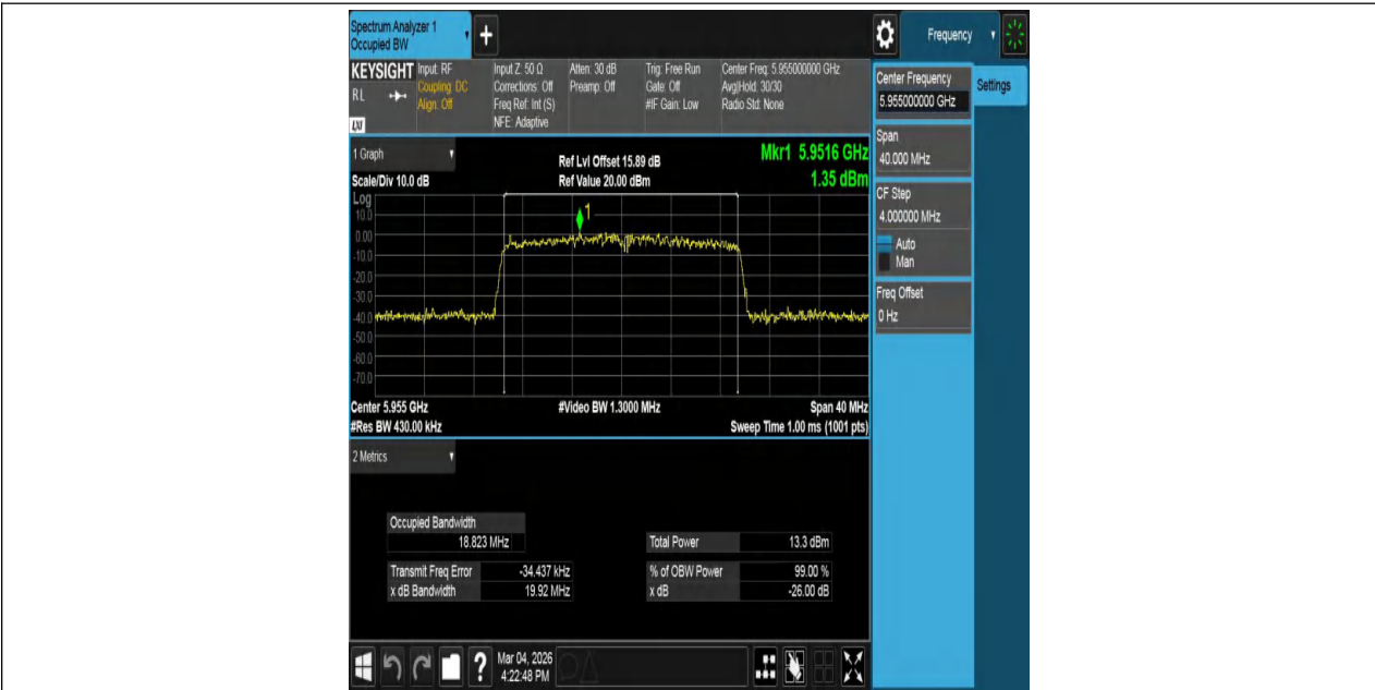
11AX20MIMO-Ant1-5955-PASS
