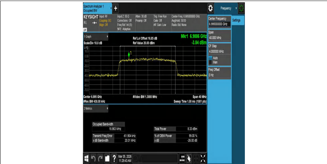
11AX20MIMO-Ant1-6995-PASS
