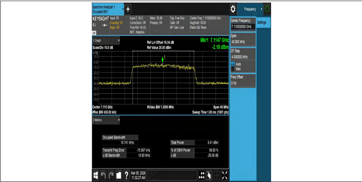
11AX20MIMO-Ant1-7115-PASS
