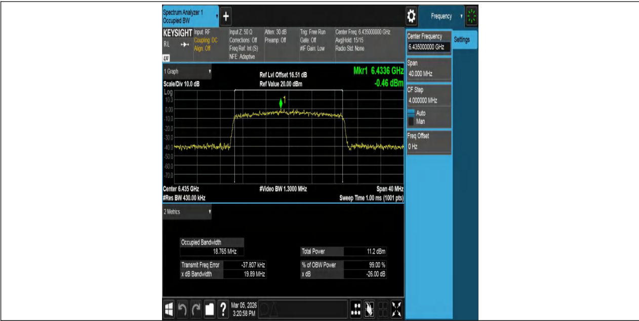
11BE20MIMO-Ant1-6435-PASS
