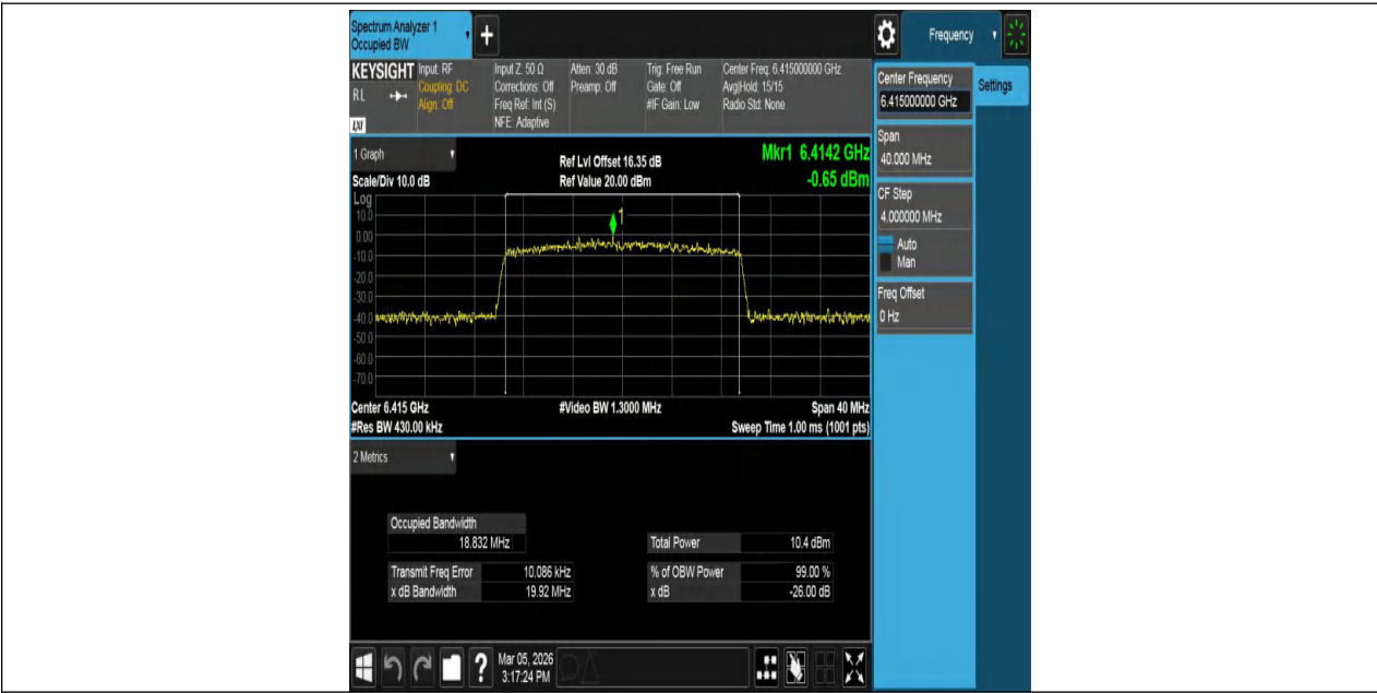
11BE20MIMO-Ant1-6415-PASS
