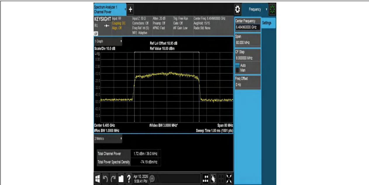
11AX40MIMO-Ant1-6485-PASS
