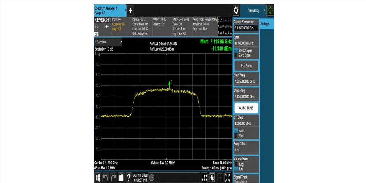
11AX20MIMO-Ant1-7115-PASS
