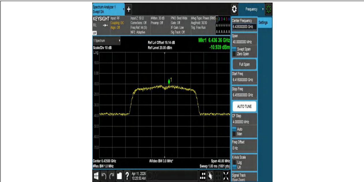
11BE20MIMO-Ant1-6435-PASS
