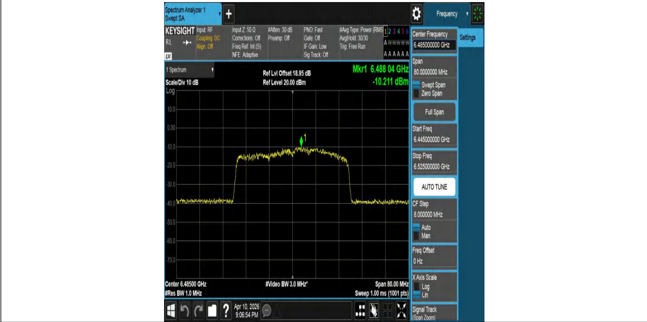
11AX40MIMO-Ant1-6485-PASS
