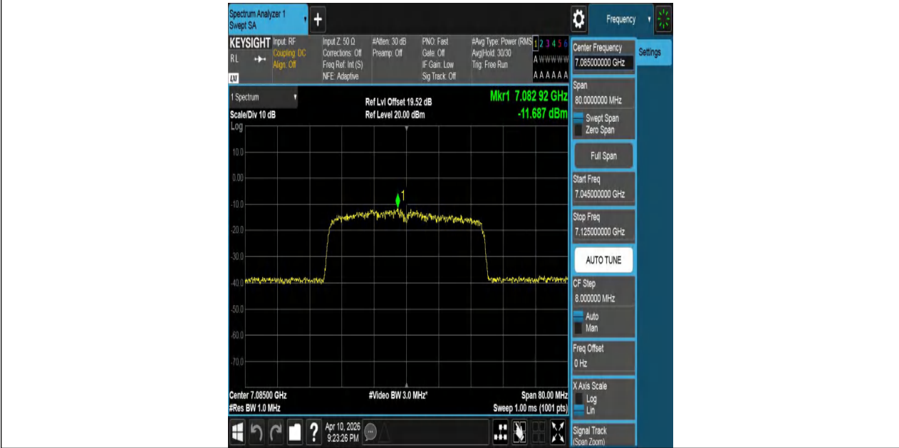
11AX40MIMO-Ant1-7085-PASS
