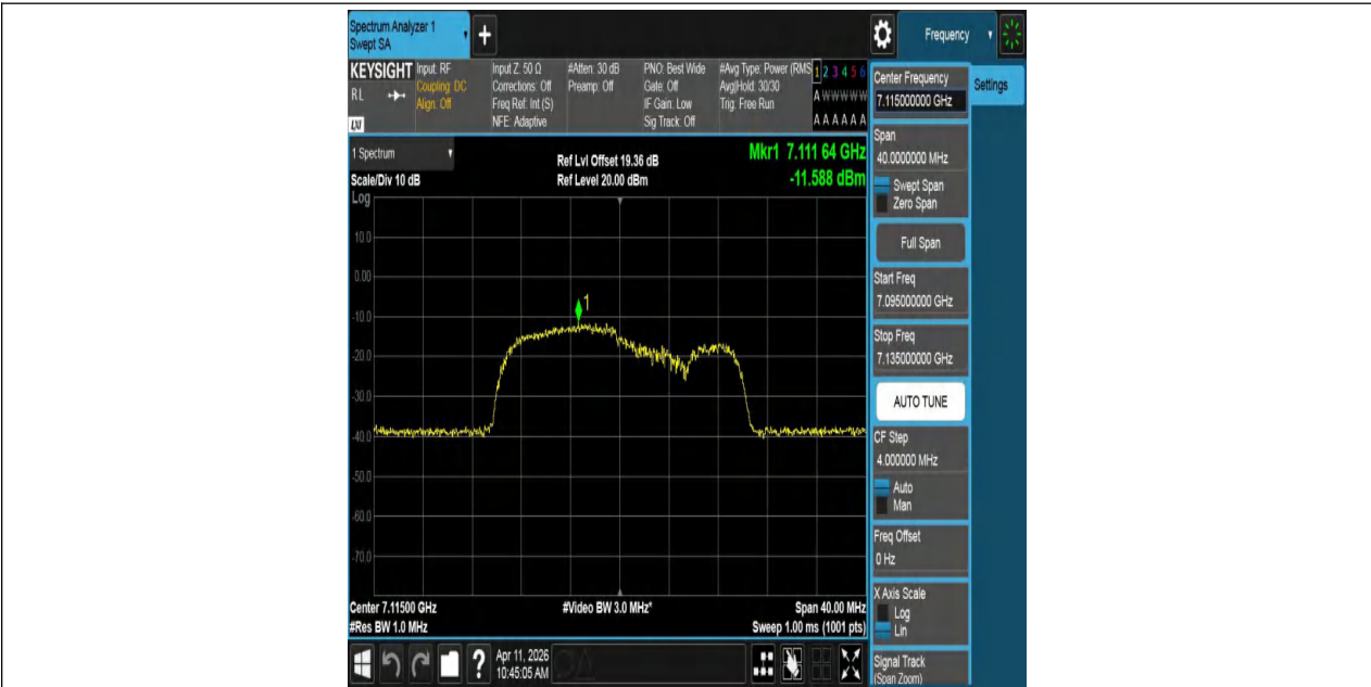
11BE20MIMO-Ant1-7115-PASS
