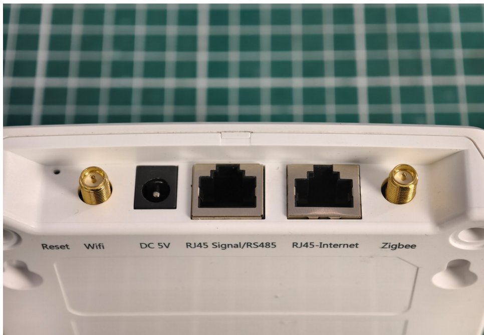
a: EUT
