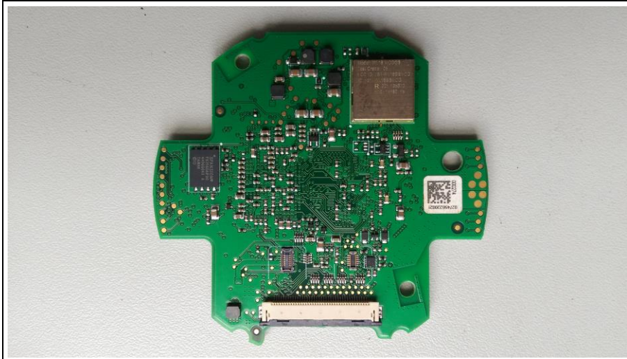
EUT PCB 1 Back
