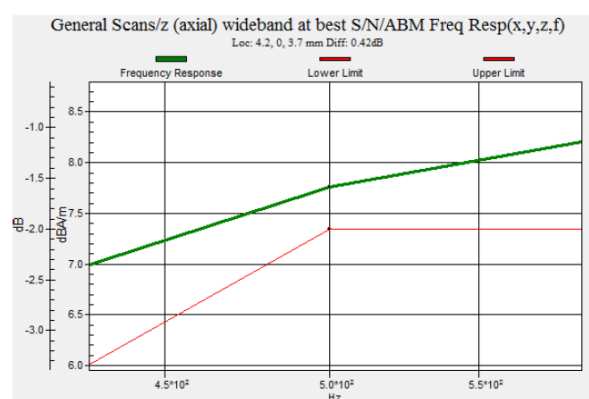
Fig. 7.6 WCDMA Band V Ch4182
