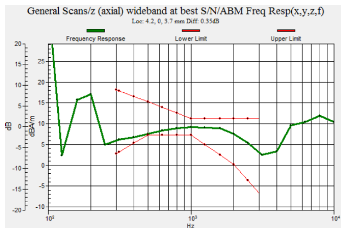
Fig. 7.11 WCDMA Band II Ch9400
