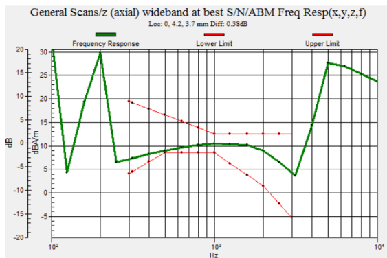
Fig 7.1 GSM850 Ch189
