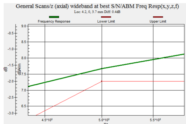
Fig. 7.8 WCDMA Band IV Ch1413
