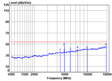
BLE_1M_TX_CH_39_Horizontal-Avg
