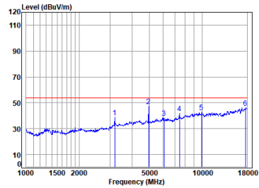
BLE_1M_TX_CH_39_Vertical-Avg
