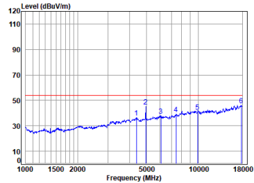
BLE_2M_TX_CH_39_Horizontal-Avg
