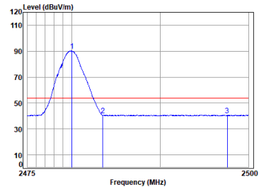
BLE_2M_TX_CH_39_Vertical-AVG
