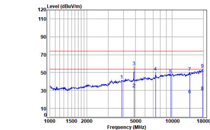
BT_DH5_TX_CH_39_Horizontal
