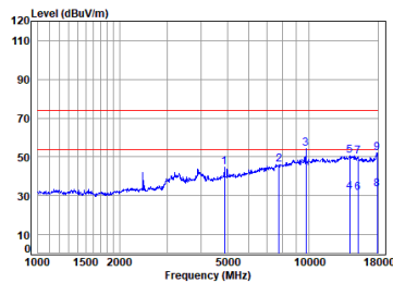
BT_2DH5_TX_CH_39_Horizontal
