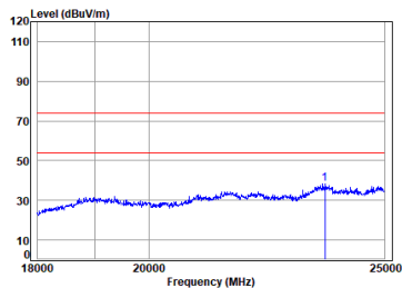
BT_2DH5_TX_CH_39_Horizontal
