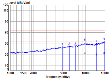
BT_DH5_TX_CH_39_Horizontal
