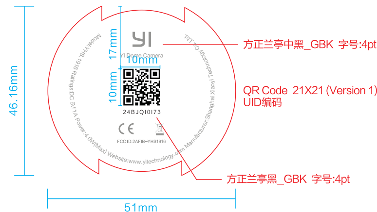
尺寸标示图:
