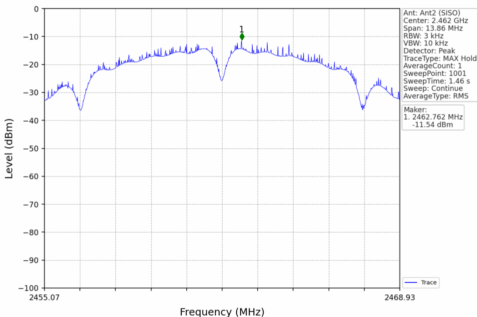
802.11b_HCH_2462MHz_Ant2 (SISO)_NTNV
