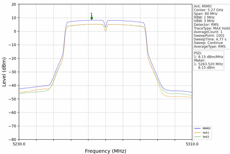
802.11n(HT40)_LCH_5270MHz_MIMO_NTNV
