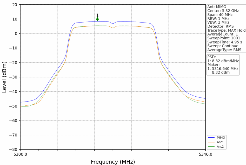
802.11n(HT20)_HCH_5320MHz_MIMO_NTNV
