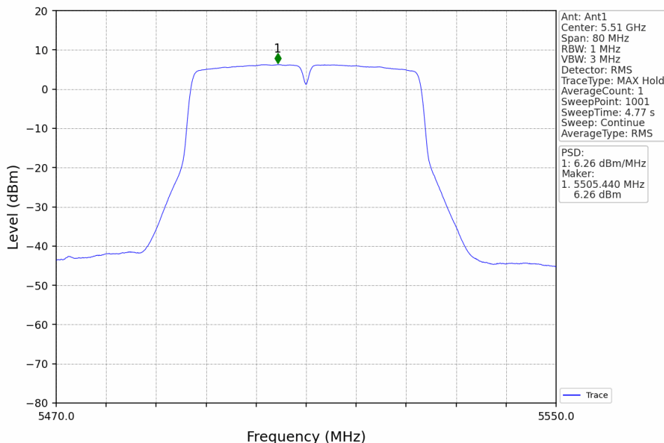
802.11n(HT40)_LCH_5510MHz_Ant1_NTNV
