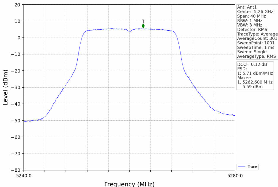
802.11n(HT20)_LCH_5260MHz_Ant1_NTNV
