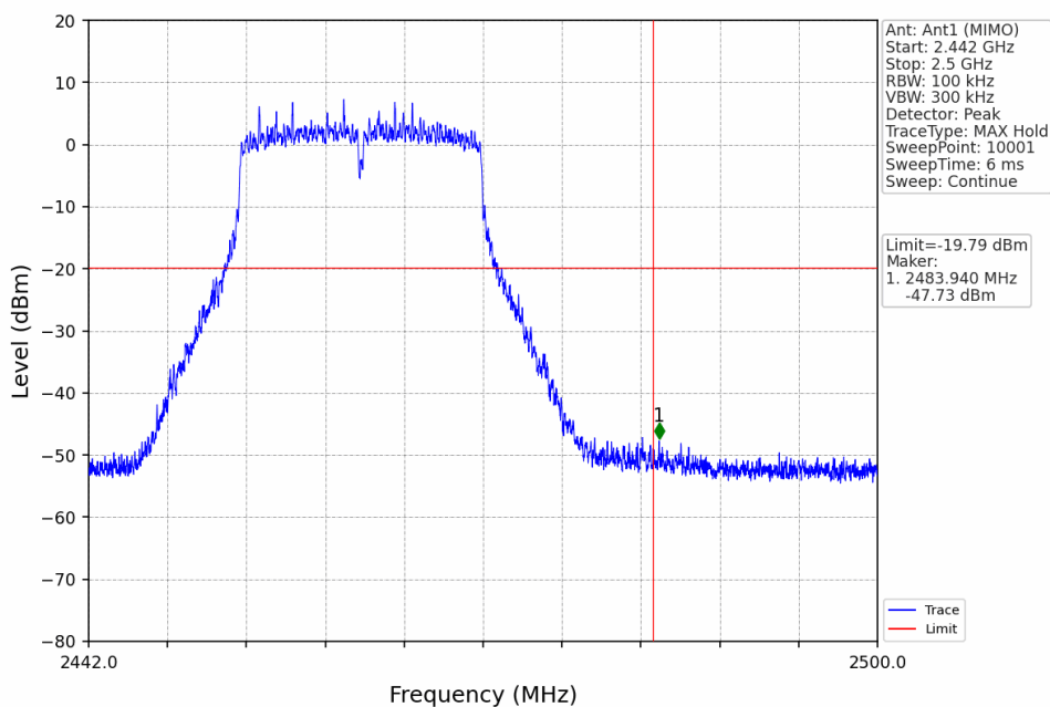
802.11n(HT20)_HCH_2462MHz_Ant1 (MIMO)_NTNV
