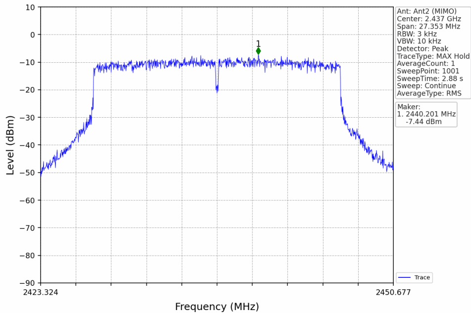
802.11ax(HEW20)_MCH_2437MHz_RU242_Left_MIMO_NTNV
