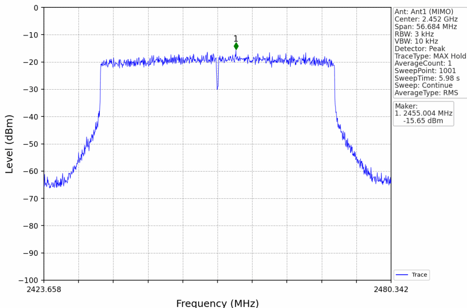
802.11ax(HEW40)_HCH_2452MHz_RU484_Left_Ant1 (MIMO)_NTNV
