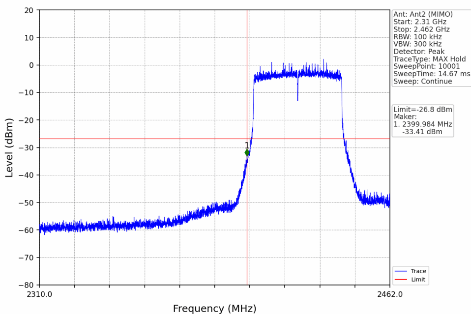
802.11ax(HEW40)_LCH_2422MHz_RU484_Left_Ant2 (MIMO)_NTNV
