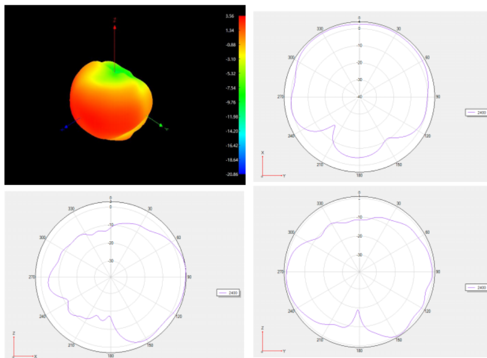
2G-1-2400MHz
