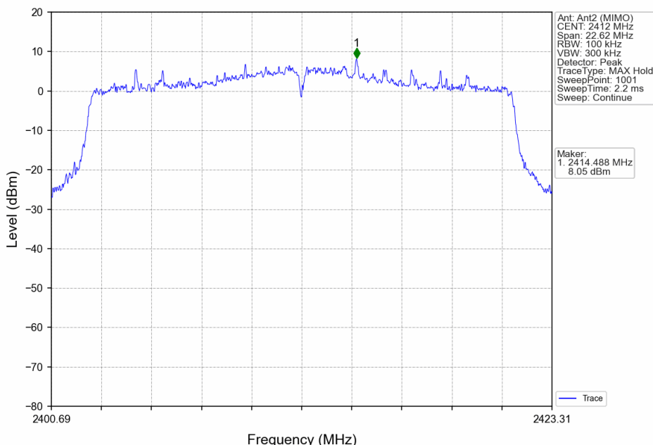
802.11ax(HEW20)_LCH_2412MHz_RU242_Left_Ant2 (MIMO)_NTNV
