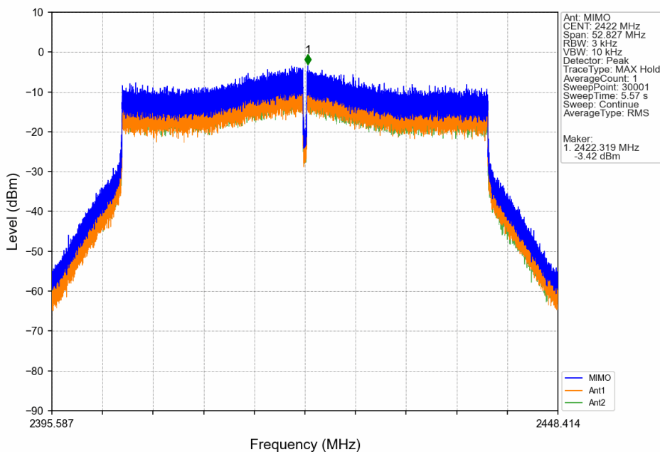
802.11be(EHT40)_LCH_2422MHz_SU_/_MIMO_NTNV
