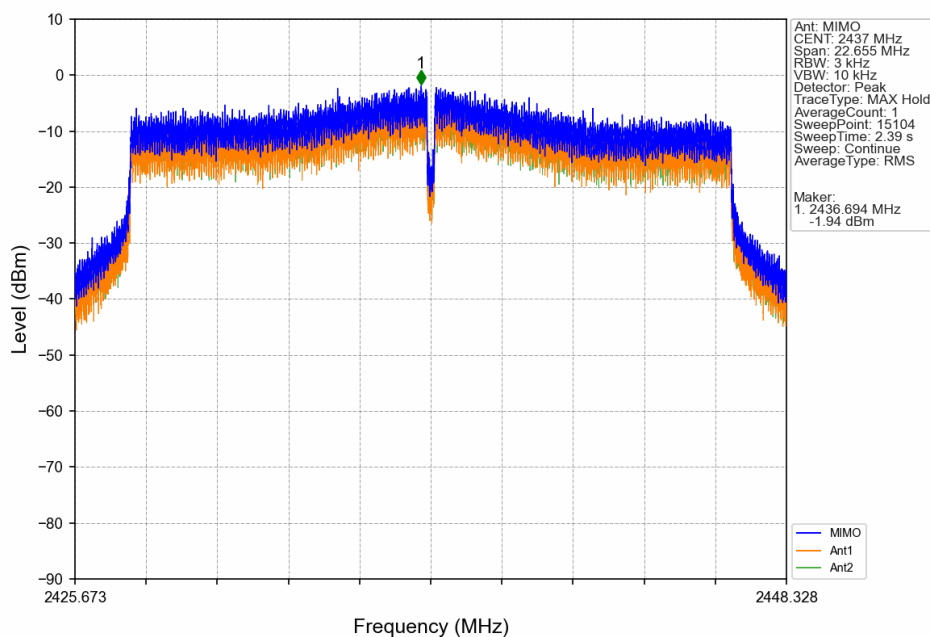
802.11be(EHT20)_MCH_2437MHz_SU_/_MIMO_NTNV
