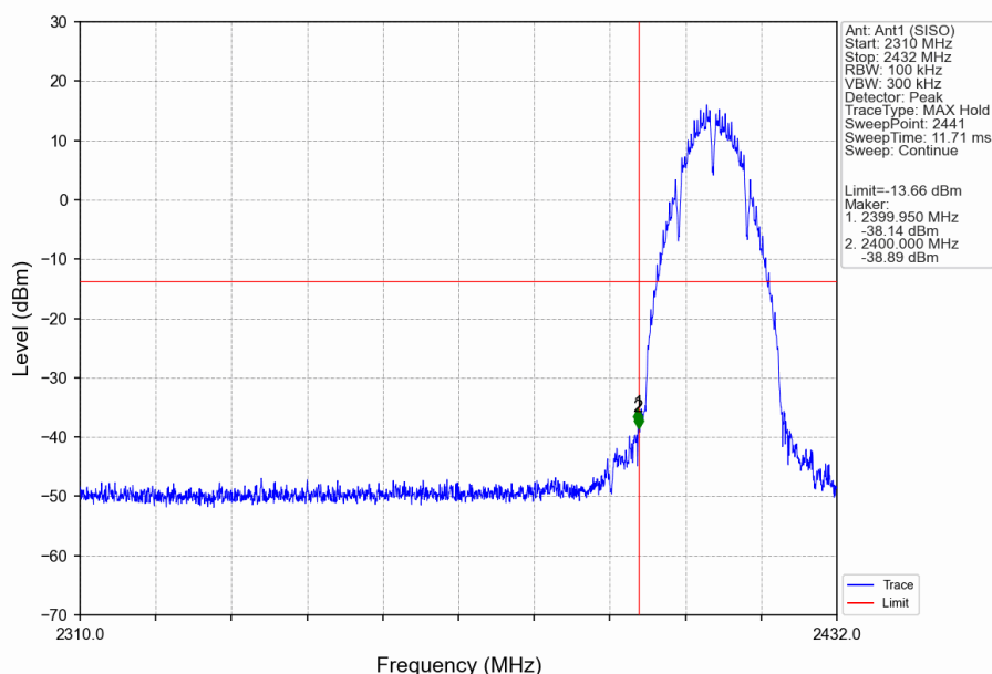
802.11b_LCH_2412MHz_Ant1 (SISO)_NTNV
