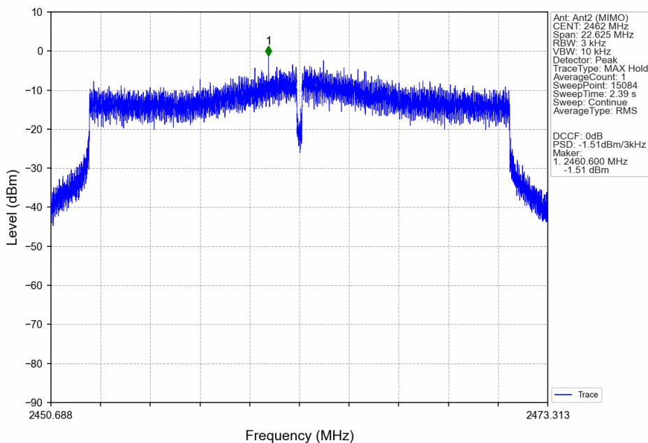
802.11be(EHT20)_HCH_2462MHz_SU_/_Ant2 (MIMO)_NTNV
