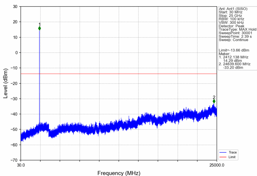
802.11b_LCH_2412MHz_Ant1 (SISO)_NTNV
