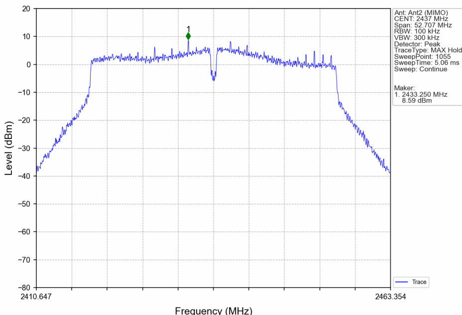
802.11n(HT40)_MCH_2437MHz_Ant2 (MIMO)_NTNV
