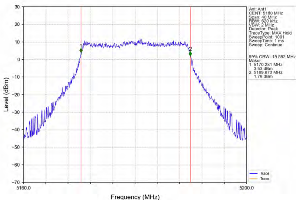
802.11be(EHT20)_LCH_5180MHz_SU_/_Ant1_NTNV
