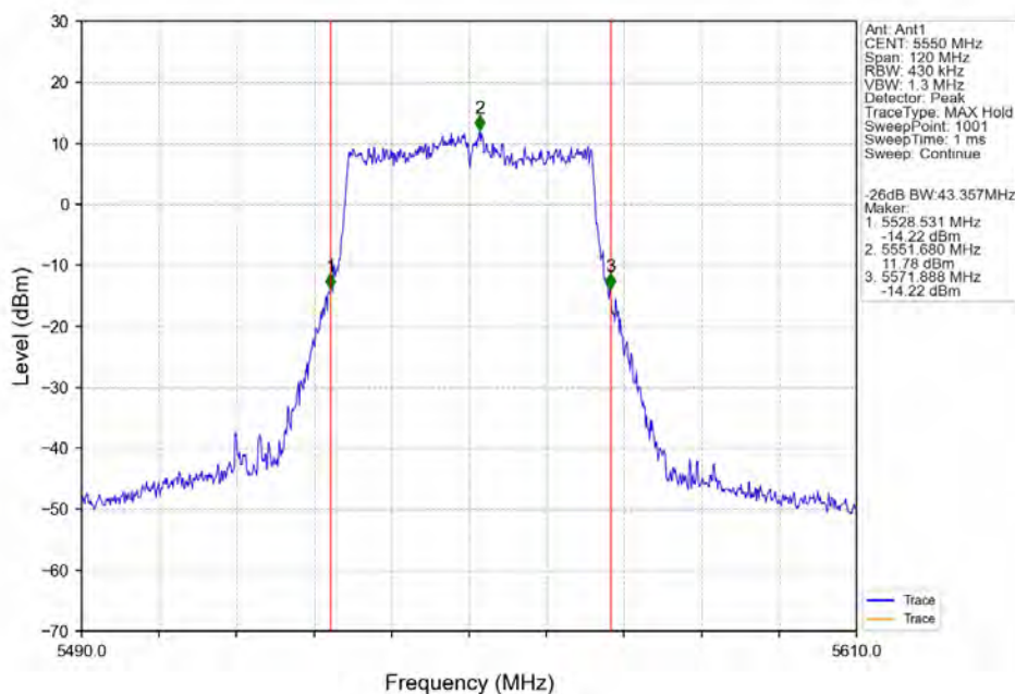
802.11be(EHT40)_MCH_5550MHz_SU_/_Ant1_NTNV
