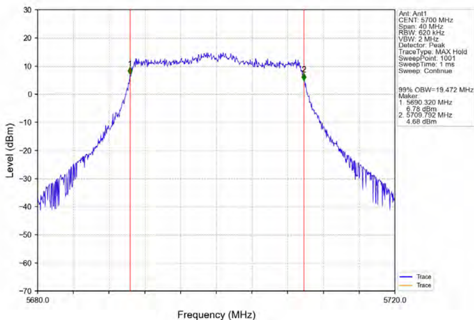
802.11be(EHT20)_HCH_5700MHz_SU_/_Ant1_NTNV
